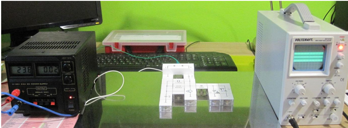
Abbildung 13: Test der Sendeeinheit 13,56 MHz
