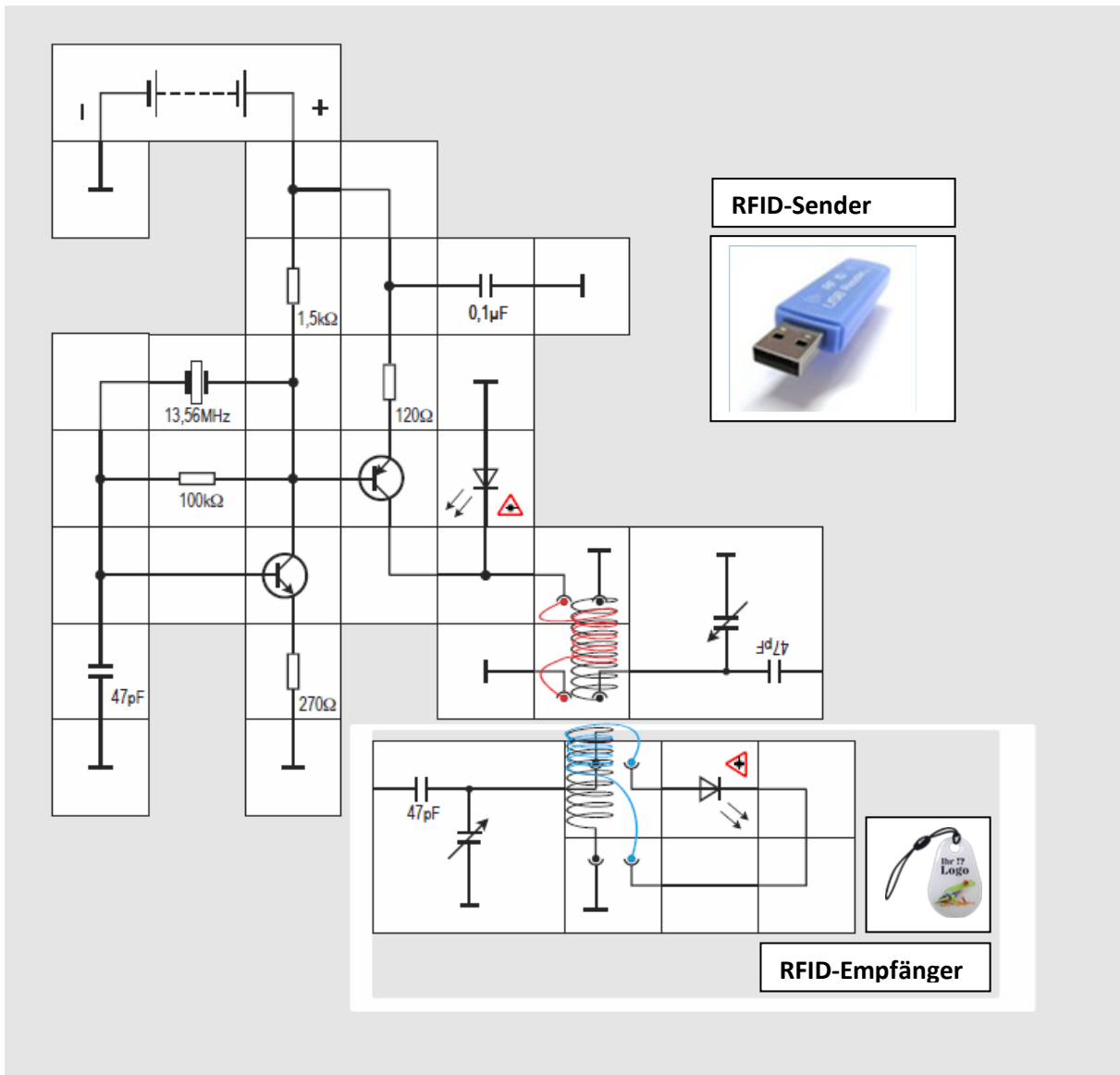
Abbildung 11: Nachweis der Energieübertragung mit dem Baukasten von Lectron
