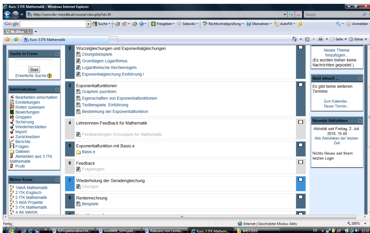
Abbildung 11: Moodle-Ansicht Mathematik
